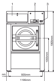
FRONTANSICHT FS 33 40 55
