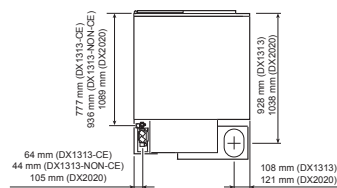
Seitenansicht DX 13/13 20/20 Gas
