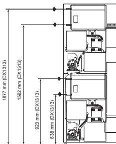
Seitenansicht DX 13/13 Dampf
