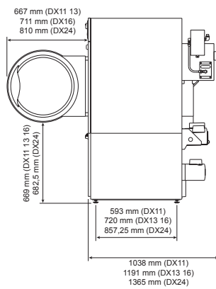
Seitenansicht DX 11 13 16 24
